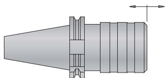
Flytande gängchuck GS/NCL - DIN 69871 A
