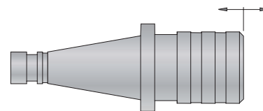
Flytande gängchuck GS/NCL - DIN 2080
