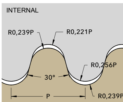
Round DIN 405
