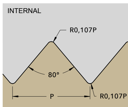
PG DIN 40430
