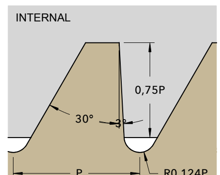
SG DIN 513
