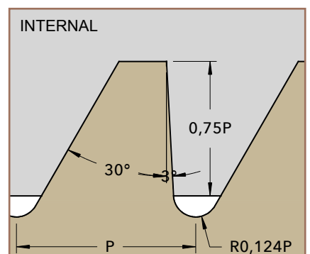
SG DIN 513
